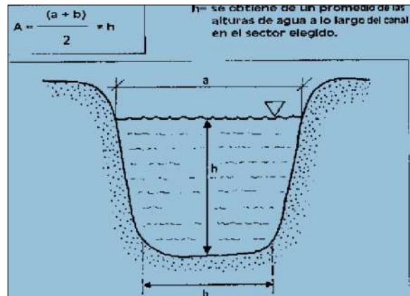
Figura 73. Se observa medida de la profundidad (h) en la sección del río Hualgayoc MP-7, para calcular el área del canal.
