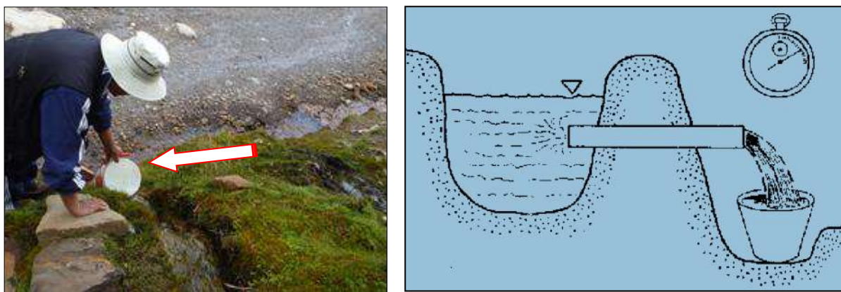
Figura 69. Medida del caudal de agua por el método volumétrico en el punto MP-4 tributario de la Bocamina la Zarza.
