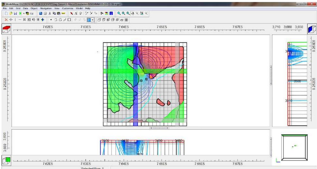
Figura 37. Superficie piezométrica de los sectores Pz-Q, Pz-S y Pz-I respectivamente, en los que se aprecia las zonas de influencia de los bombeos. Se han representado los vectores de velocidad.
