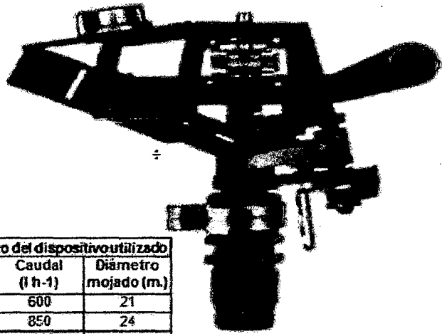
Figura 1. Características del aspersor
