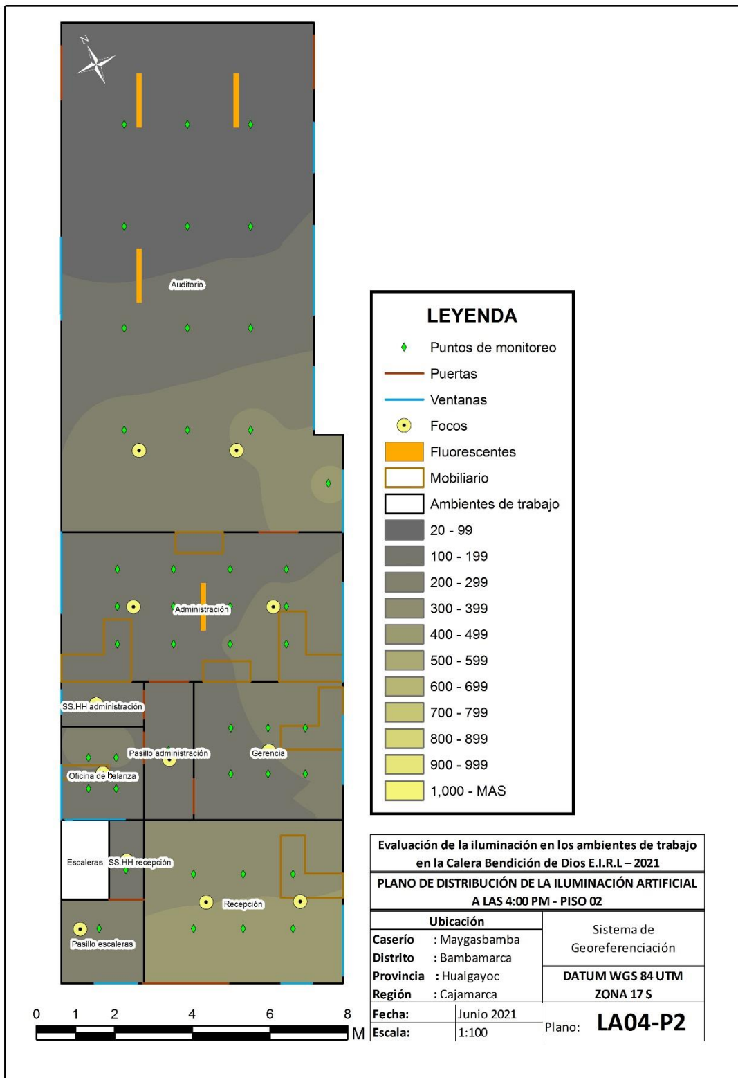
Figura 13 - Plano de distribución de la iluminación artificial a las 4:00 pm – Piso 02
