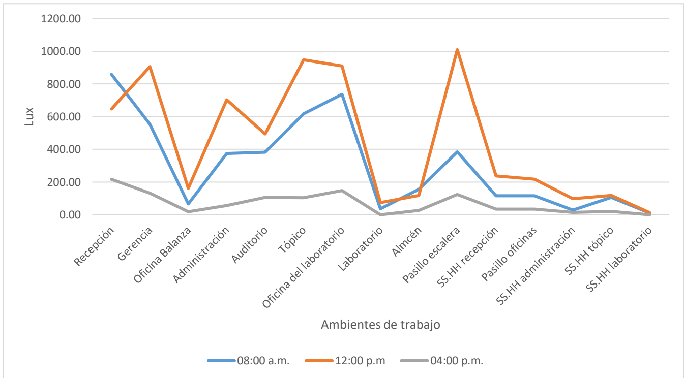
Figura 4 - Niveles de iluminación natural de los ambientes de trabajo a las 8:00 a.m., 12:00 p.m. y 4:00 p.m.
