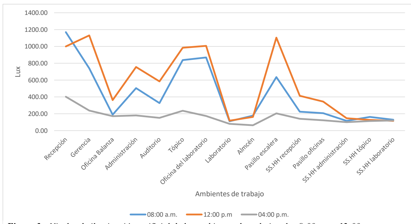
Figura 3 - Niveles de iluminación artificial de los ambientes de trabajo a las 8:00 a.m., 12:00 p.m. y 4:00 p.m.
