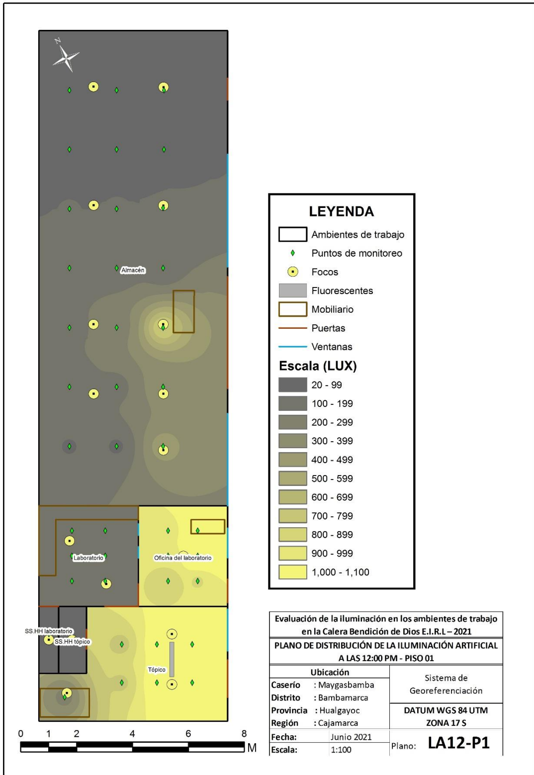
Figura 6 - Plano de distribución de la iluminación artificial a las 12:00 pm – Piso 01
