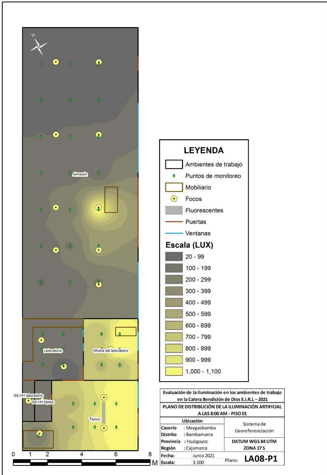
Figura 5 - Plano de distribución de la iluminación artificial a las 8:00 am – Piso 01
