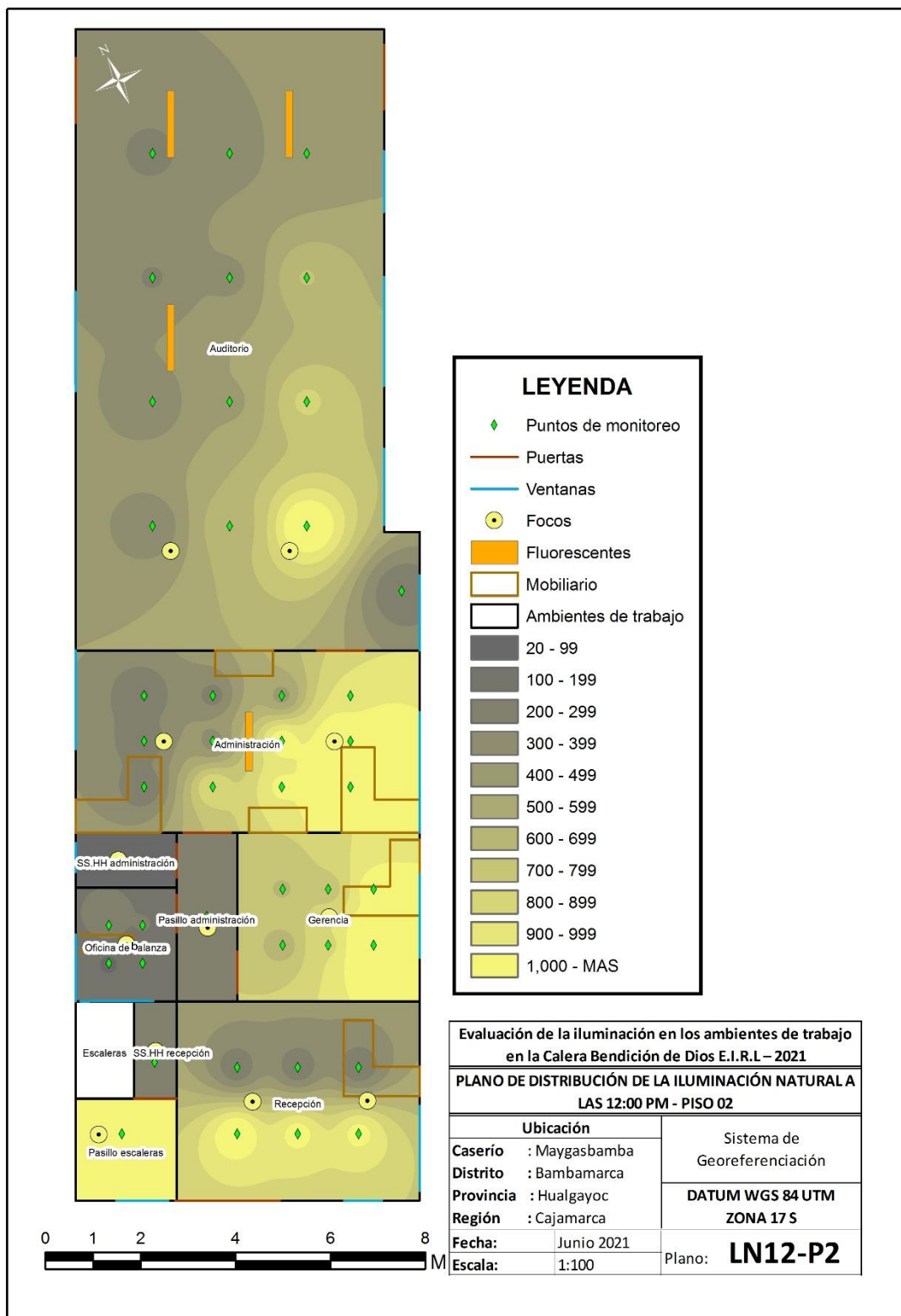
Figura 15 - Plano de distribución de la iluminación natural a las 12:00 pm – Piso 02
