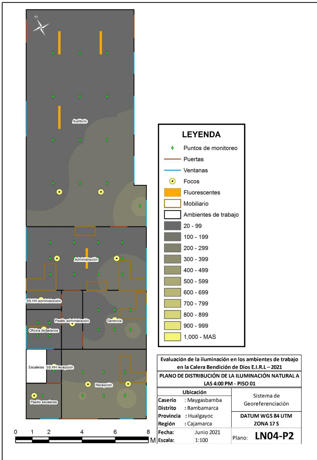
Figura 16 - Plano de distribución de la iluminación natural a las 4:00 pm – Piso 02
