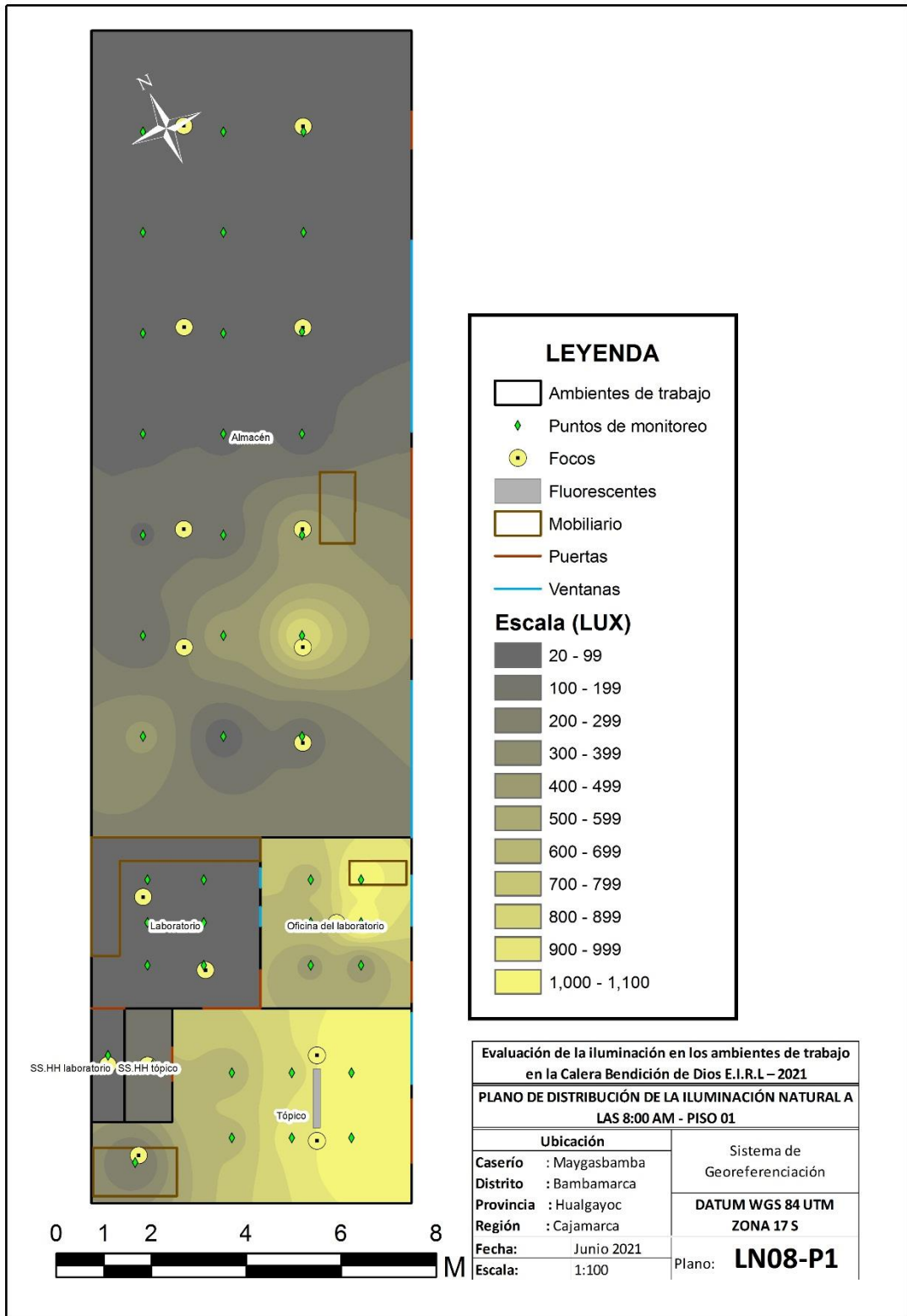
Figura 8 - Plano de distribución de la iluminación natural a las 8:00 am – Piso 01
