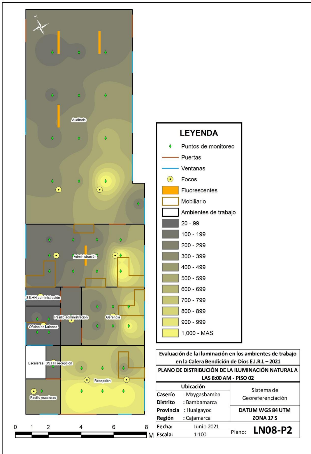
Figura 14 - Plano de distribución de la iluminación natural a las 8:00 am – Piso 02
