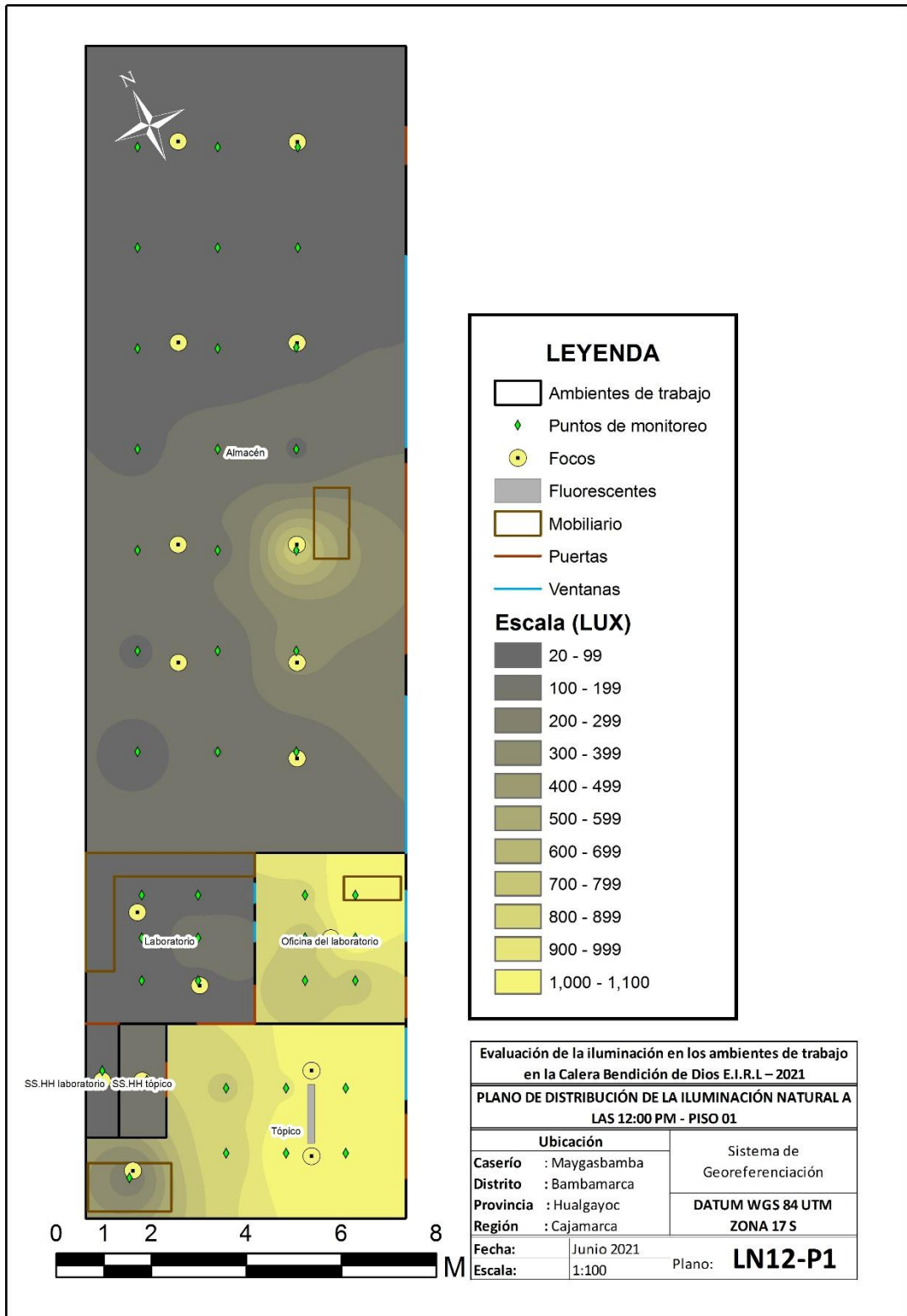
Figura 9 - Plano de distribución de la iluminación natural a las 12:00 pm – Piso 01
