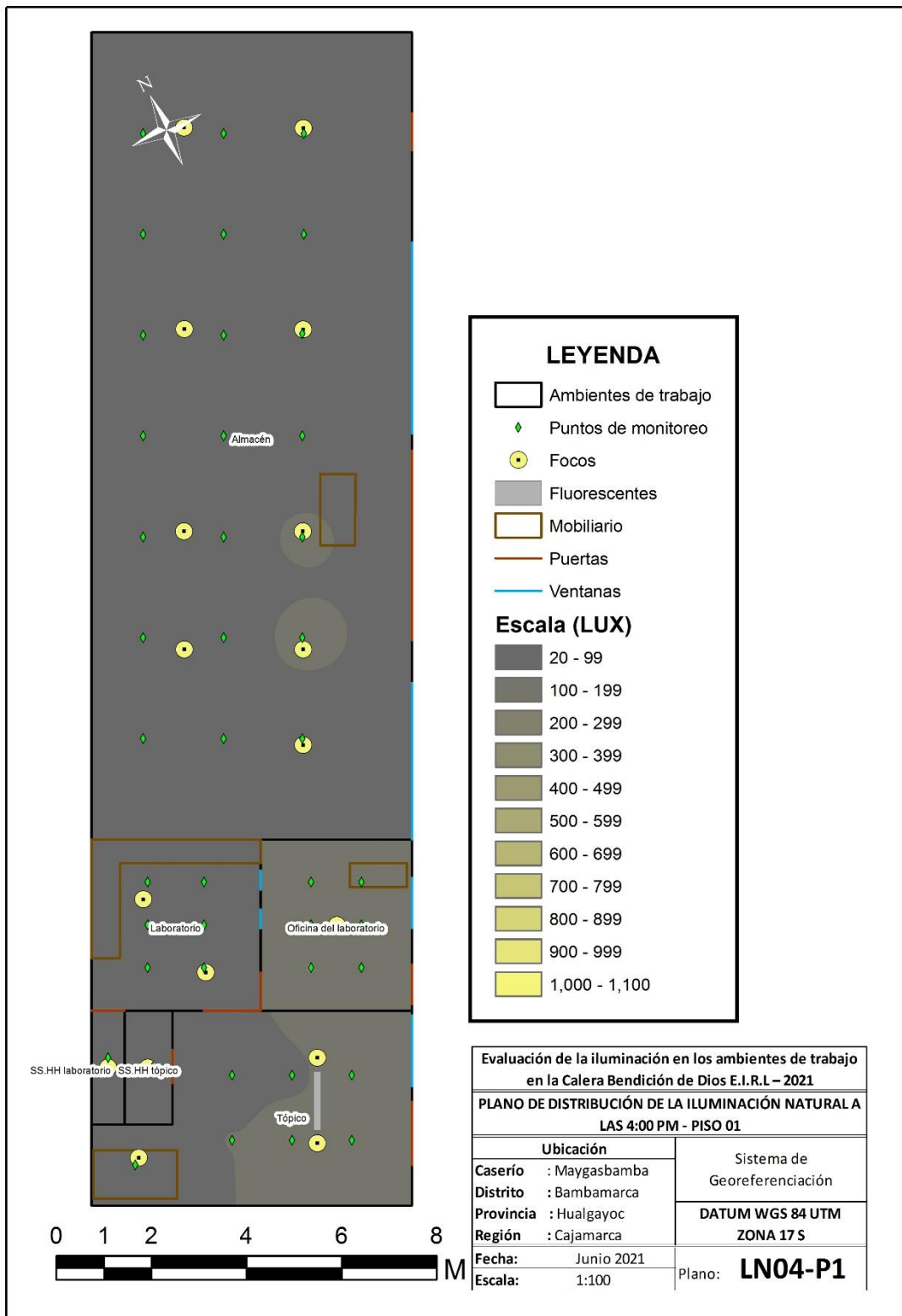
Figura 10 - Plano de distribución de la iluminación natural a las 4:00 pm – Piso 01
