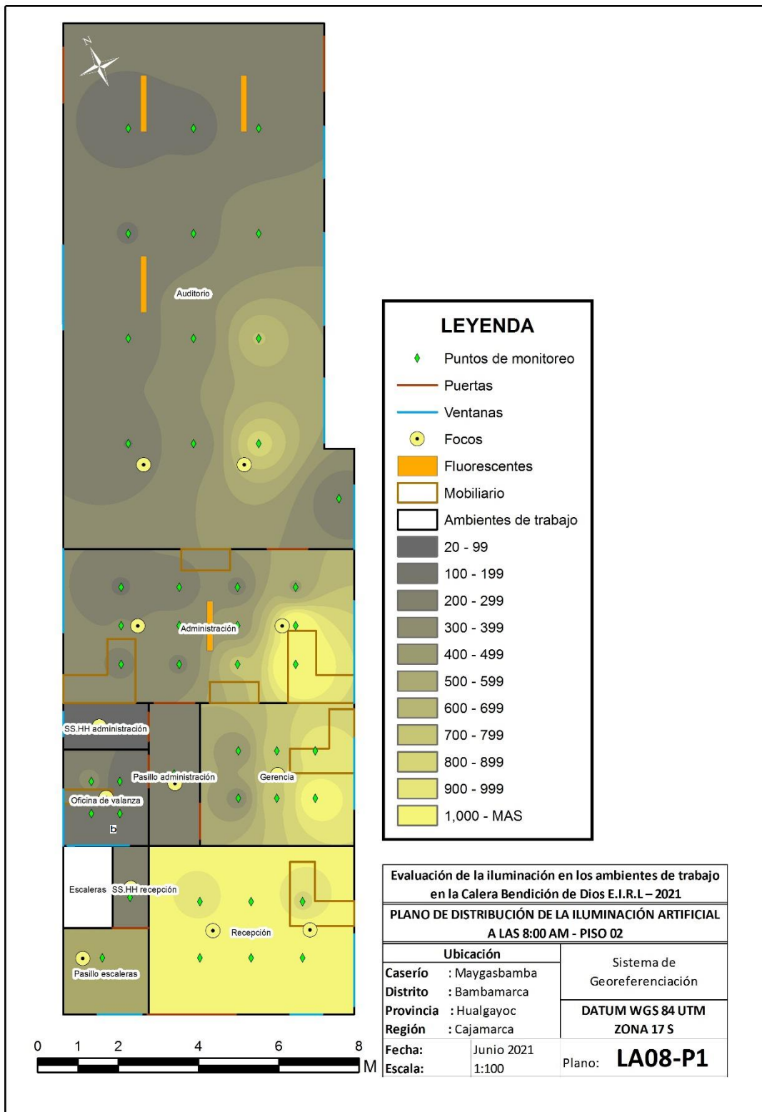
Figura 11 - Plano de distribución de la iluminación artificial a las 8:00 am – Piso 02
