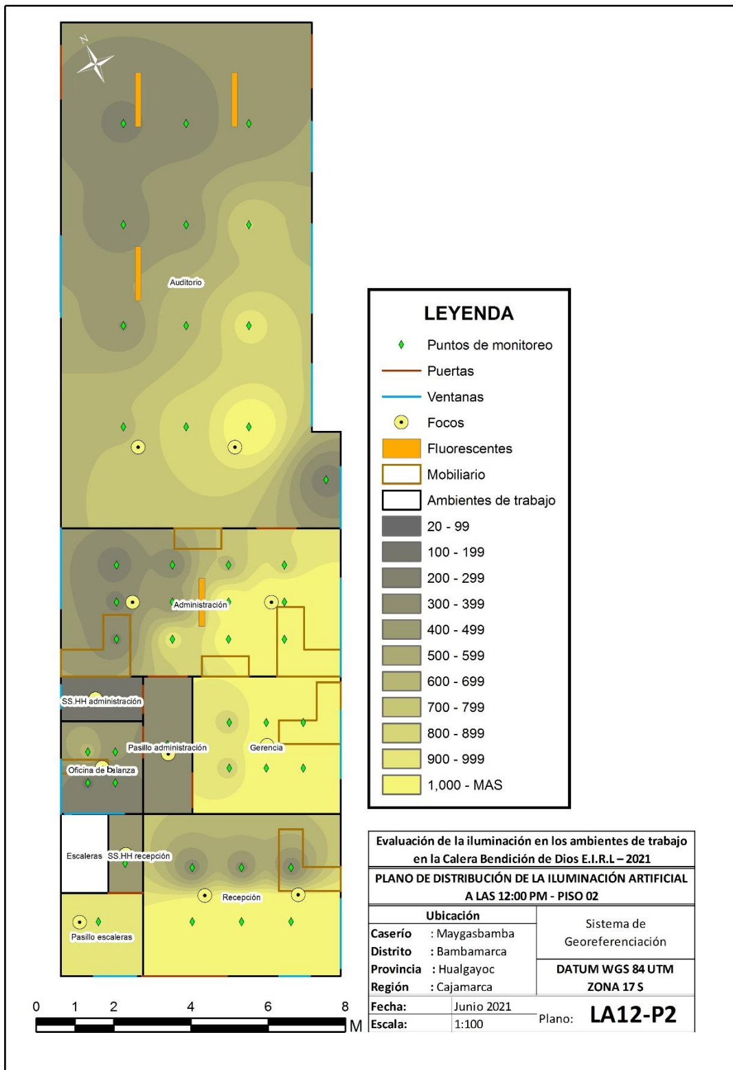
Figura 12 - Plano de distribución de la iluminación artificial a las 12:00 pm – Piso 02
