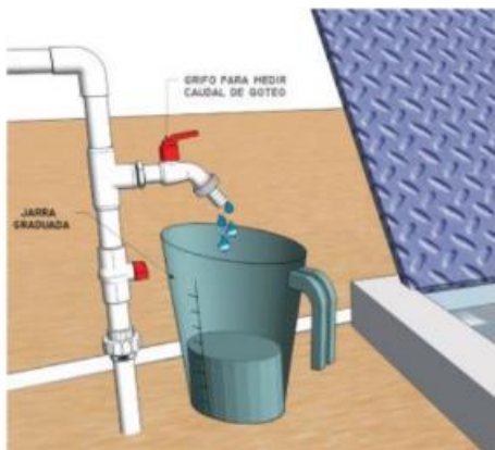
Figura 7: Caudal de goteo
