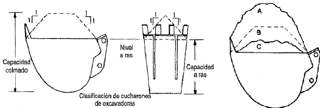
Figura 2.6. Capacidad del cucharón.
