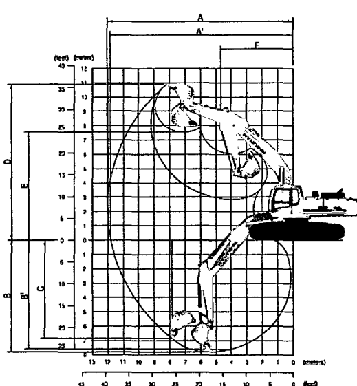
Figura 2.8. Gamma de trabajo excavadora Hyundai Robex 500LC
