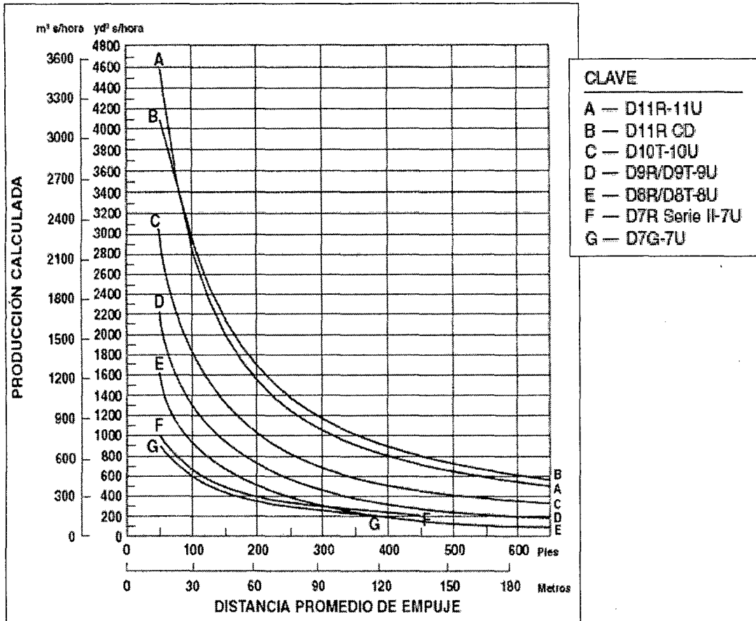
Figura 2.3. Abaco para calcular rendimientos máximos teóricos tractor de orugas.
