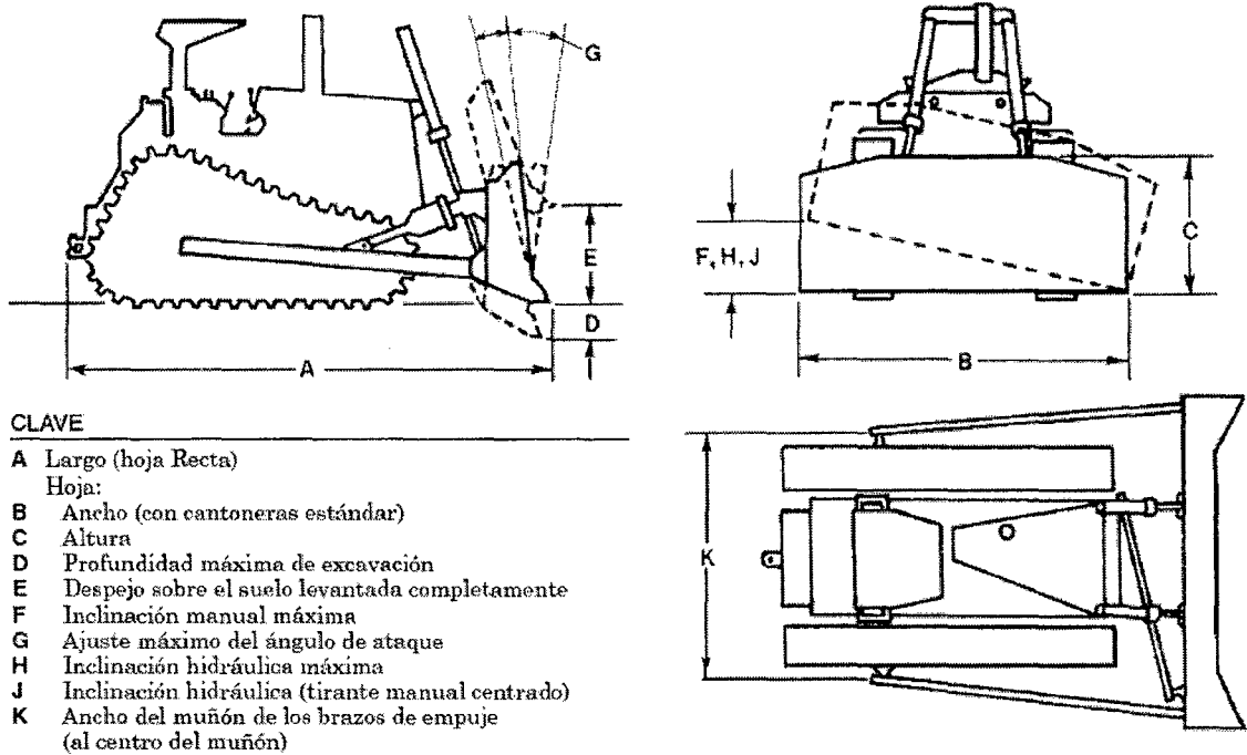
Figura 2.4. Dimensiones del tractor usado.
